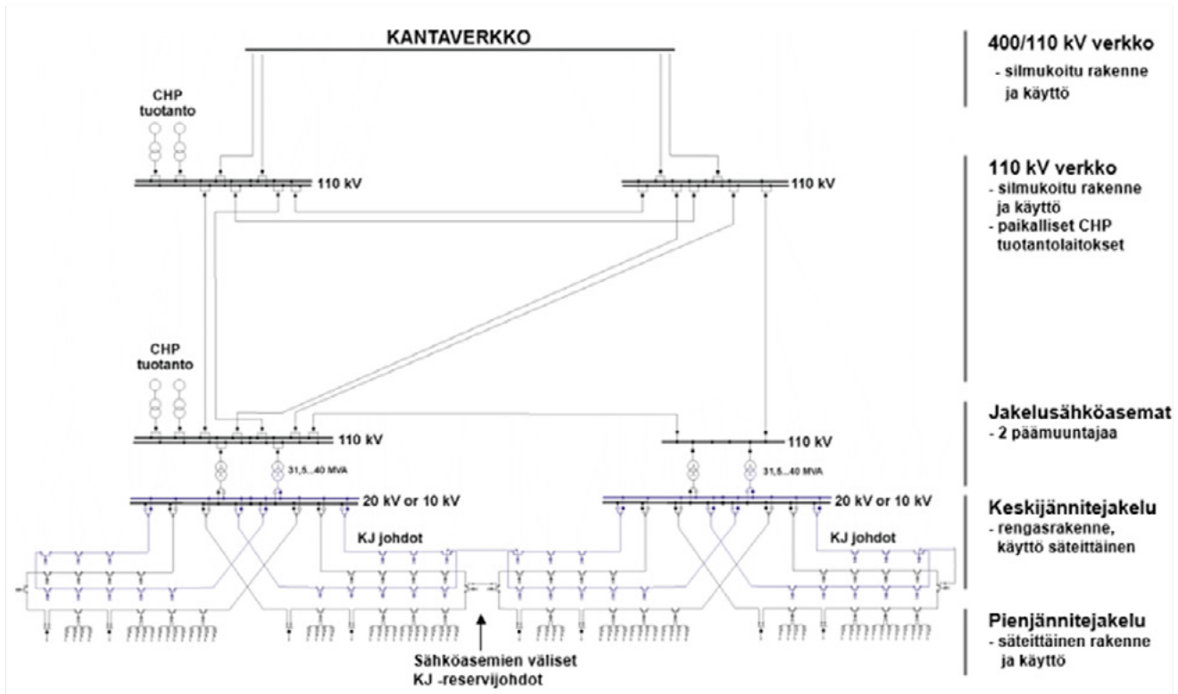
Kuva 15. Helsingin sähköjakeluverkon perusrakenne
