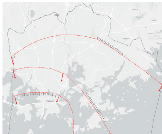
Kuva 19. Helsingin 110 kV verkon siirtorajapinnat
